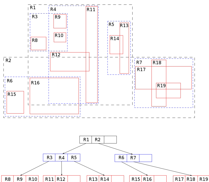
Figure 4. Exemple de segmentation de plan par arbre-R
